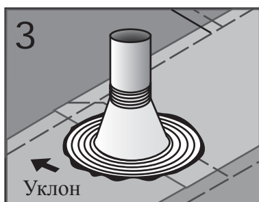
Битумно-полимерный компаунд
