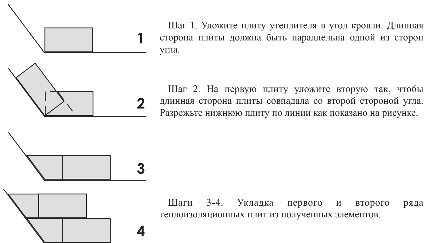
Рис. 13. Раскрой и расположение теплоизоляционных плит в не прямых углах кровли.
