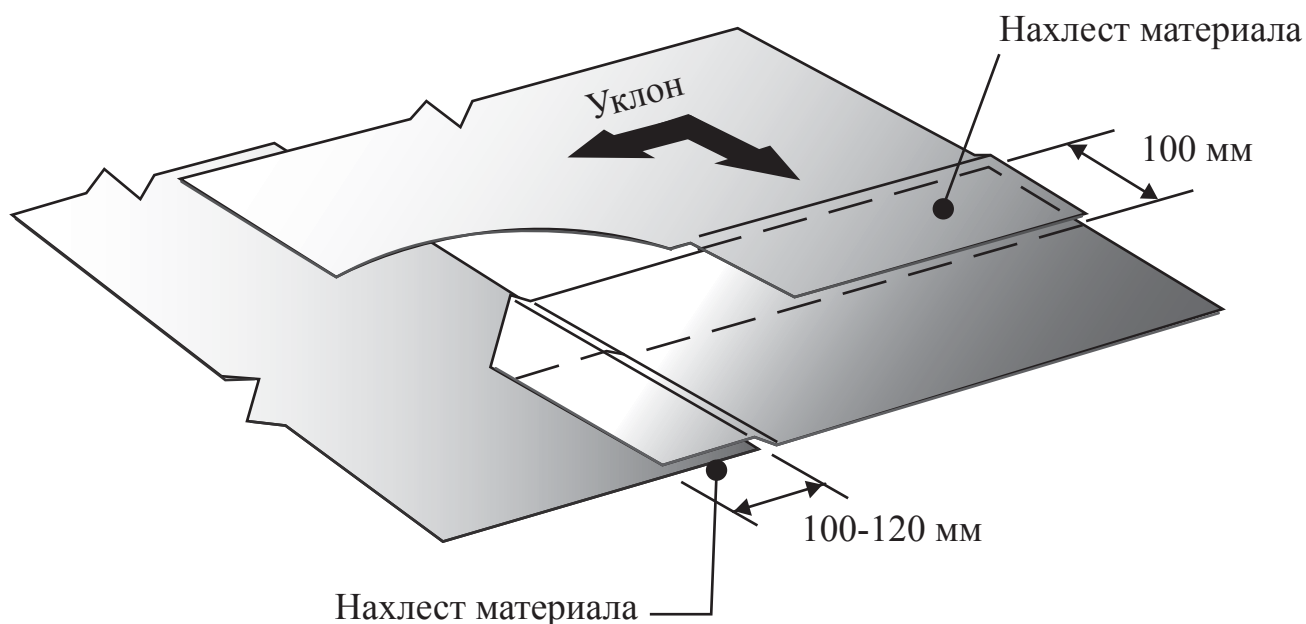
Рис. 17. Нахлесты полотнищ рулонного материала.
