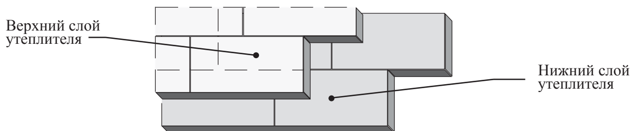
Рис. 12. Смещение плит верхнего и нижнего слоев при укладке.
