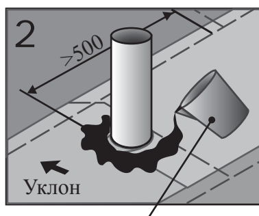
Битумно-полимерный компаунд
