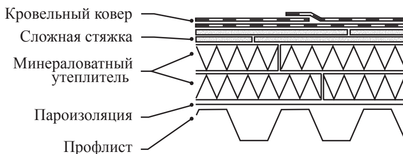
Рис. 4. Гидроизоляционный ковер по сборной стяжке.
